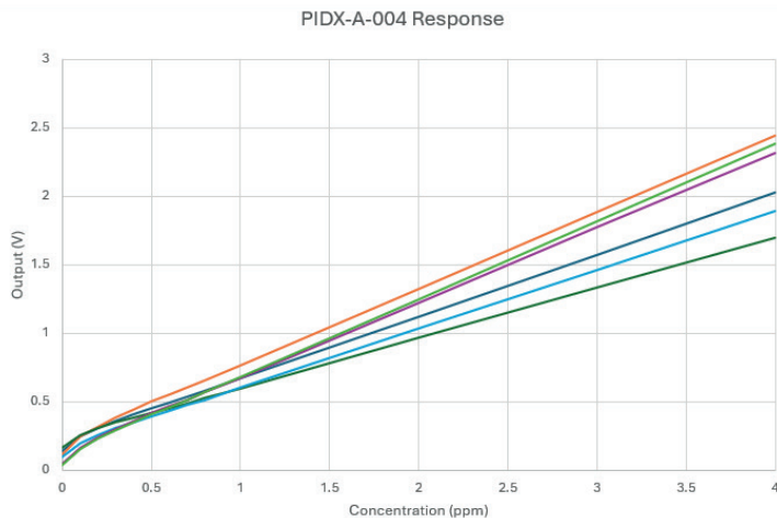
Fig. 1 PIDX-A-004线性度 (0-4 ppm)
