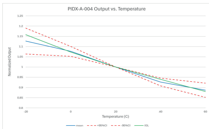
Fig. 2 灵敏度温度特性
